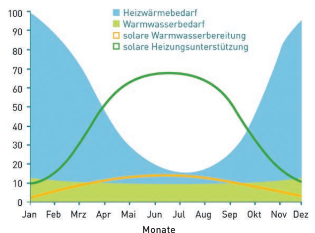
Abbildung 53: Sonnenwärmeangebot und Wärmebedarf im Bestandsgebäude
