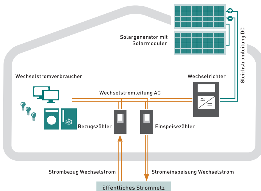
Abbildung 34: Aufbau einer netzgekoppelten Photovoltaikanlage
