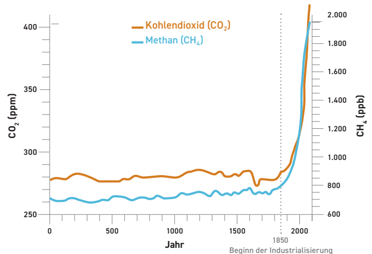
Abbildung 3: Entwicklung der Konzentration wichtiger Treibhausgase in der Atmosphäre, 0 bis 2020
