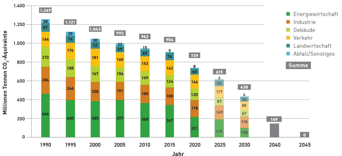
Abbildung 7: Treibhausgasemissionen in Deutschland – bisherige Entwicklungen und Ziele
