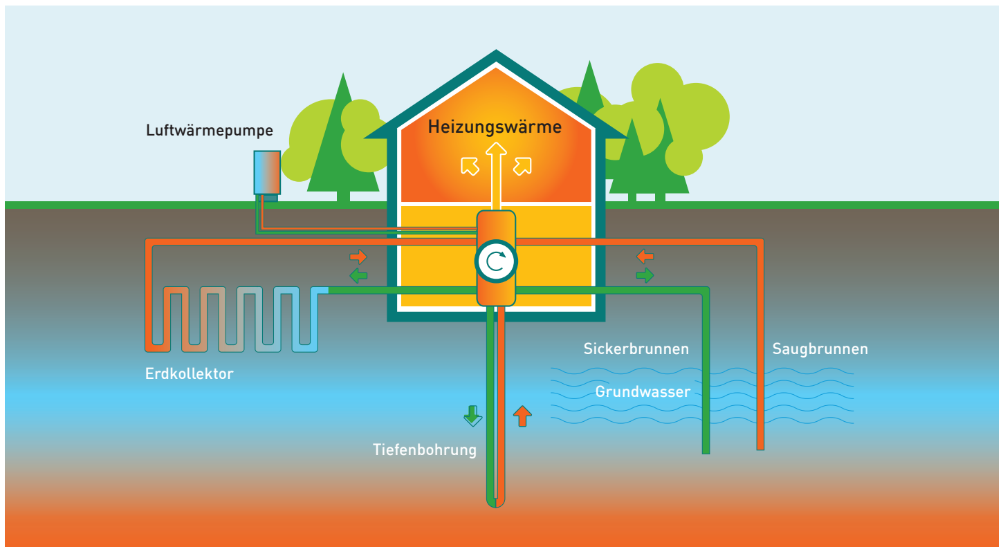
Abbildung 47: Nutzung verschiedener Wärmequellen durch Wärmepumpen
