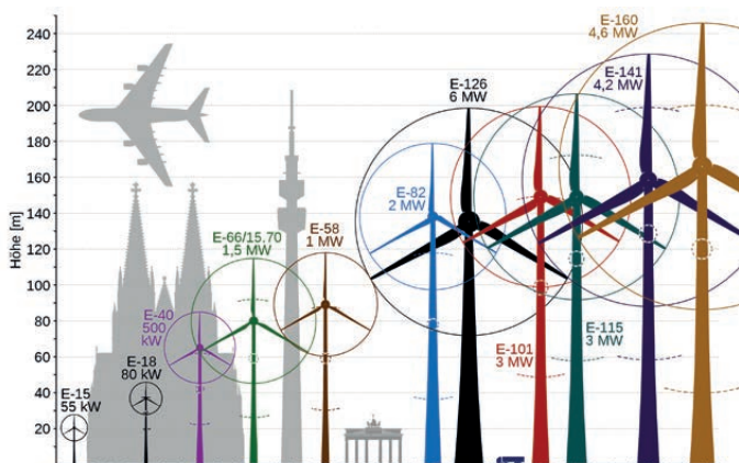
Abbildung 19: Größenentwicklung der Windenergieanlagen des Anlagenherstellers Enercon
