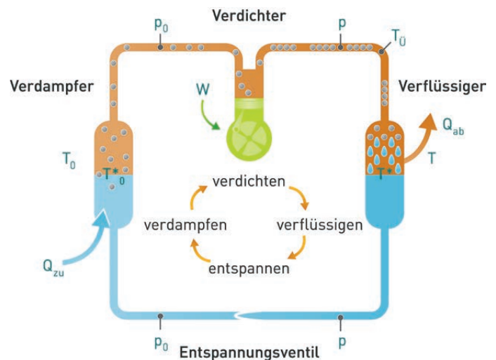
Abbildung 46: Funktionsprinzip einer Wärmepumpe
