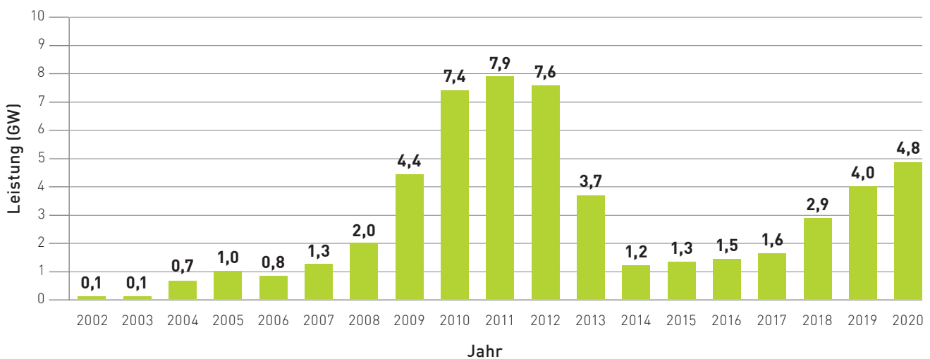
Abbildung 30: Photovoltaik Netto-Zubau installierter Nennleistung in Deutschland
