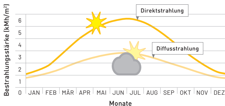
Abbildung 36: Direkt- und Diffusstrahlung im Jahresverlauf
