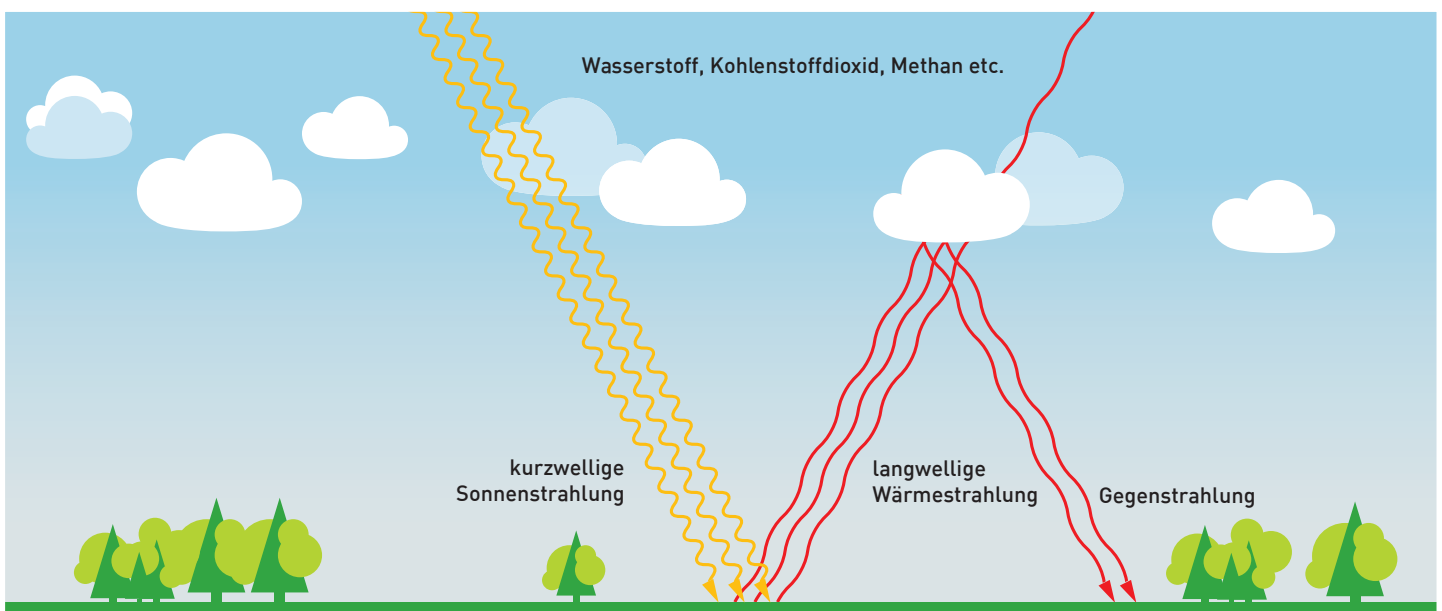
Abbildung 4: Darstellung des natürlichen Treibhauseffektes
